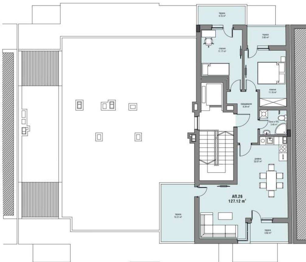
РАЗПРЕДЕЛЕНИЕ кота +17.50
